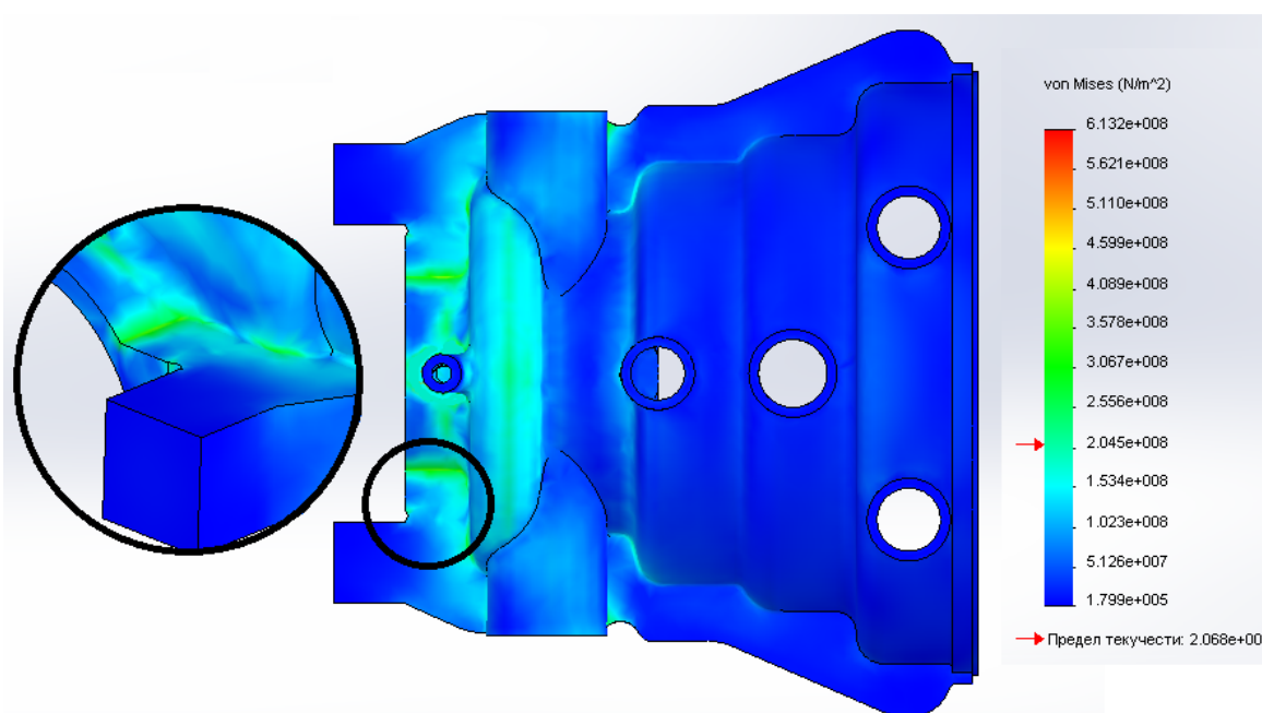
Рис. 3 – НДС корпуса ЦСД при пуске из НС-1 в момент времени 3400 сек
